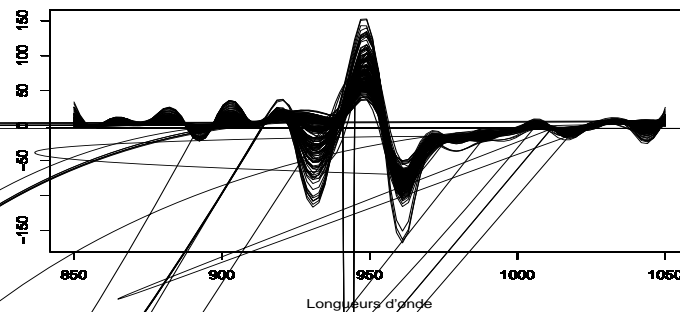
FIG. 2 – Les 215 dérivées seconde des courbes spectrométriques
