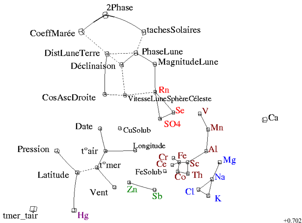
Figure 8 : iconographie des corrélations totales, au seuil 0.25 Pour les campagnes MIDLANTE, RIFT et GATE Traits pleins : corrélations > 0 ; Traits pointillés : corrélations < 0
