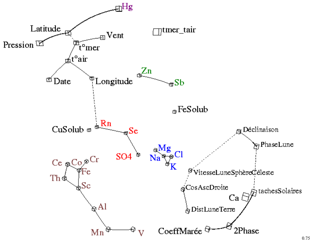
Figure 9 : corr/MagnitudeLune, au seuil 0.25
